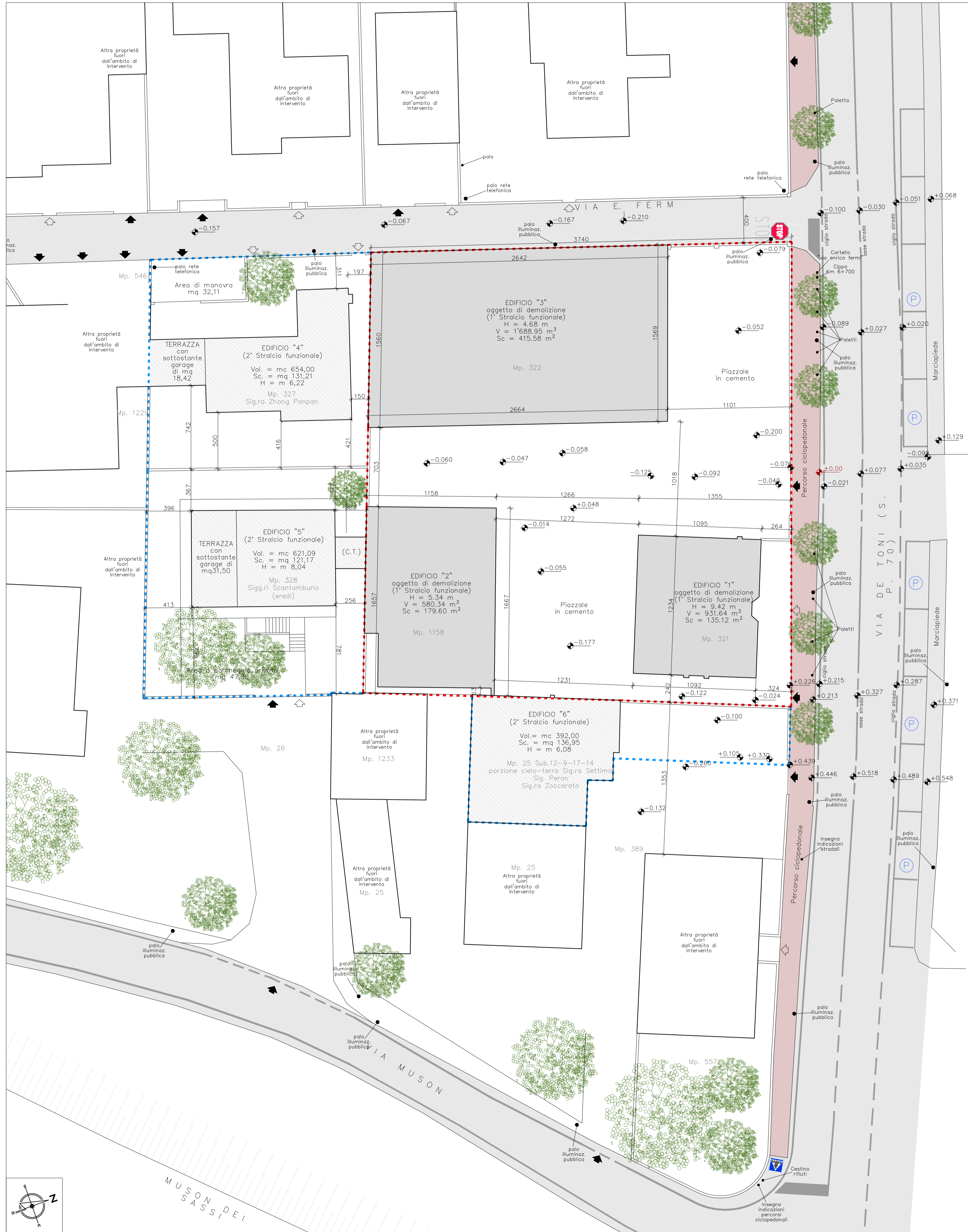
PLANIMETRIA DELLO STATO DI FATTO CON RILIEVO PLANIALTIMETRICO E CONI VISUALI
