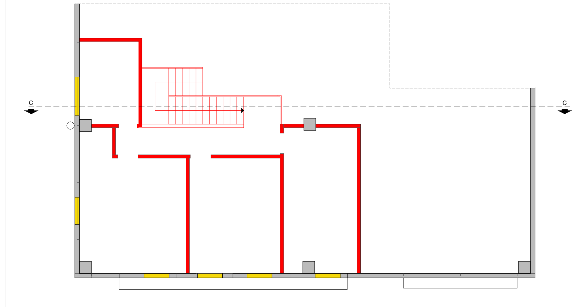
PIANO PRIMO scala 1:100
