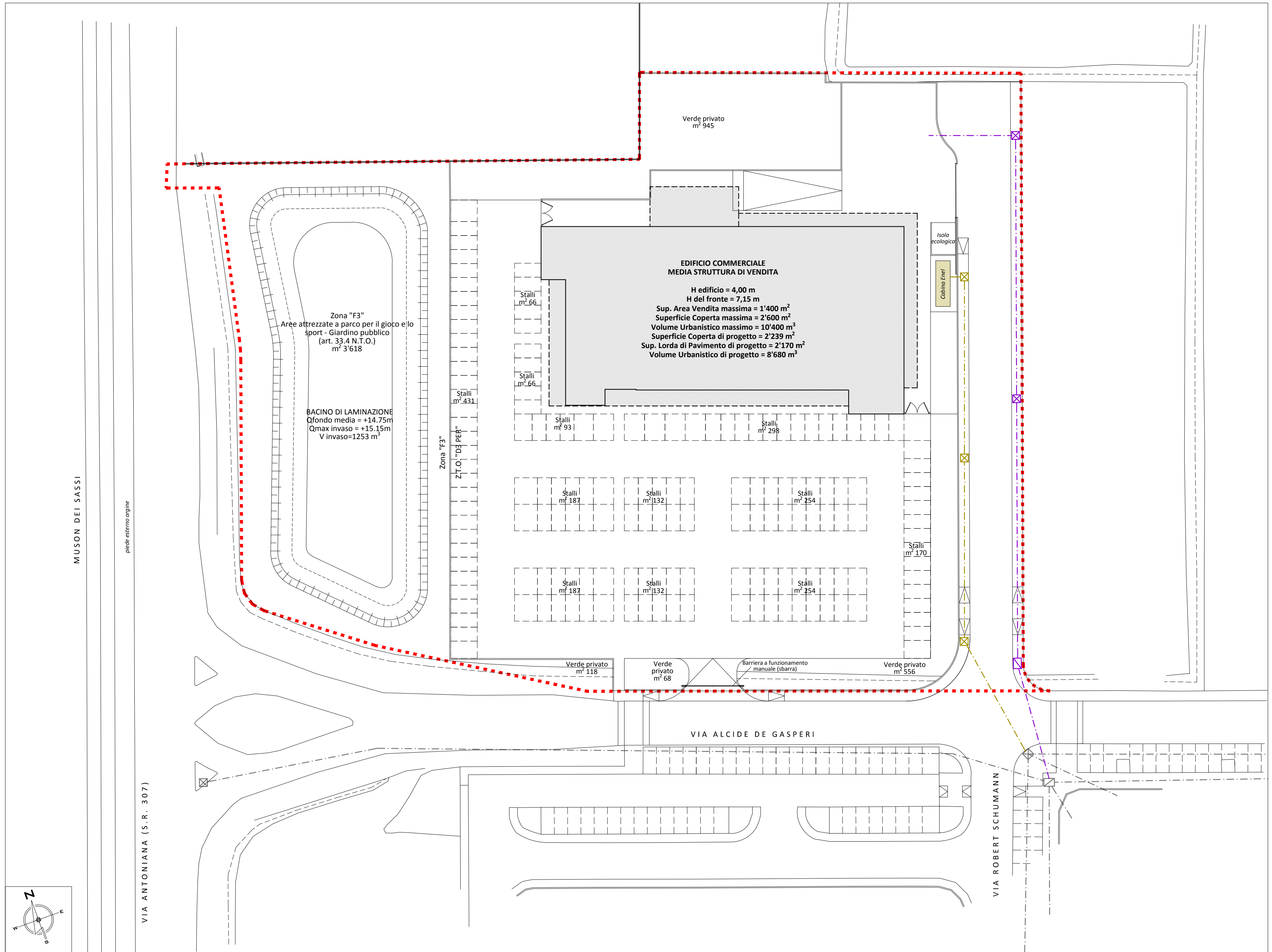
PLANIMETRIA DI PROGETTO CON SOTTOSERVIZI
