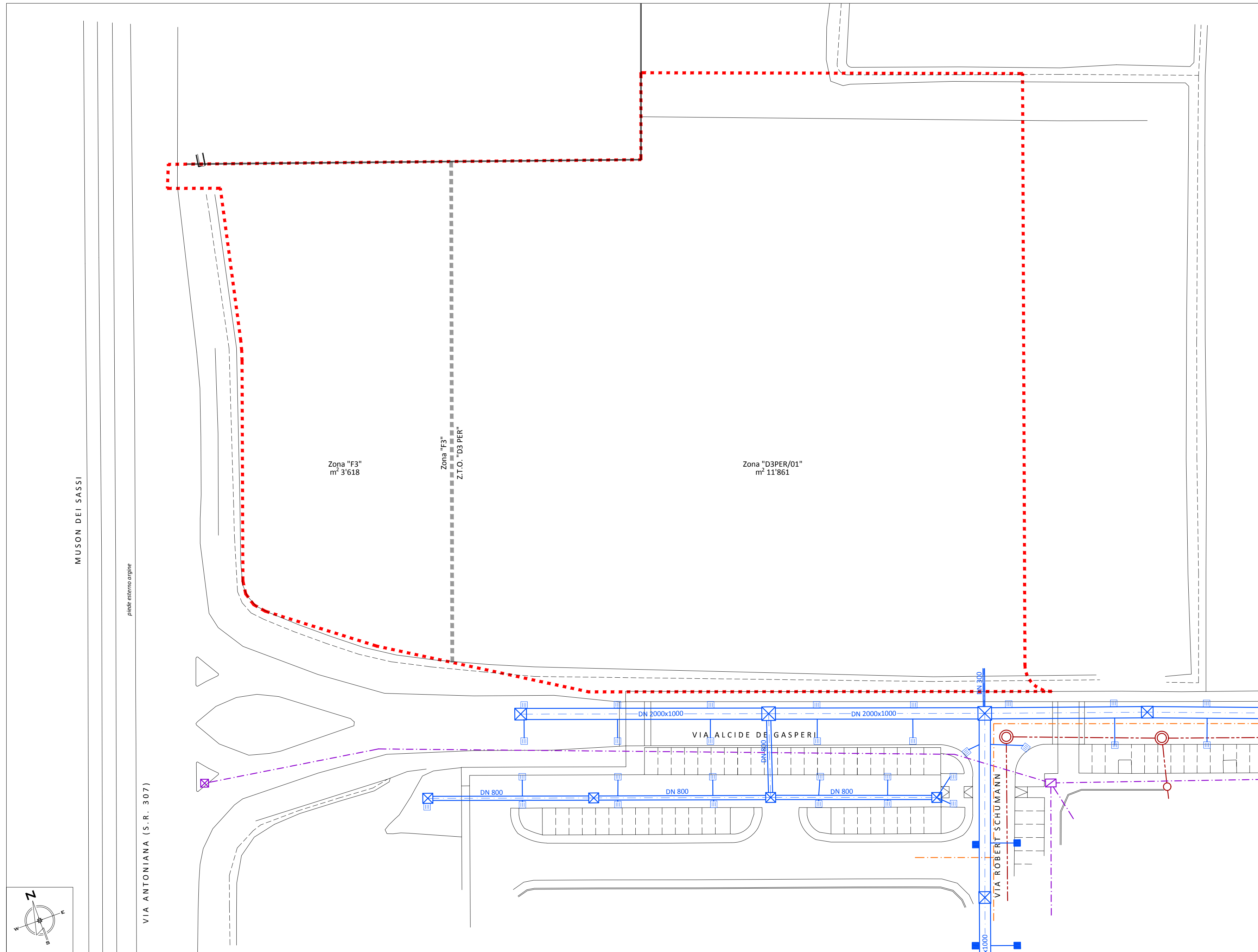
PLANIMETRIA DELLO STATO DI FATTO CON SOTTOSERVIZI
